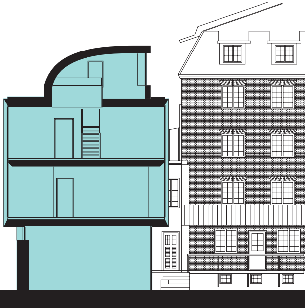
SEKTION SEDD MOT NORR
