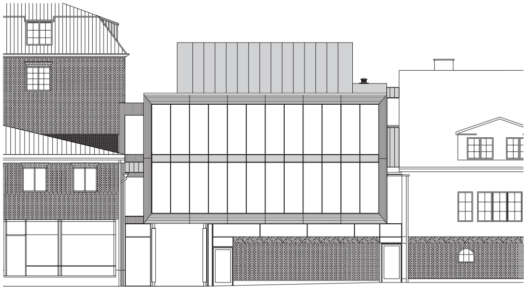
FASAD MOT VÄSTER, VÄSTERGATAN
