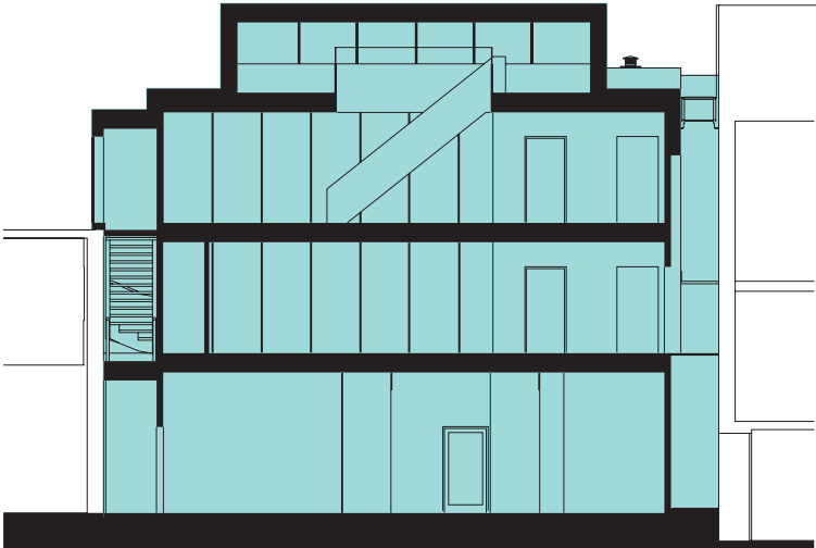
SEKTION SEDD MOT VÄSTERGATAN
