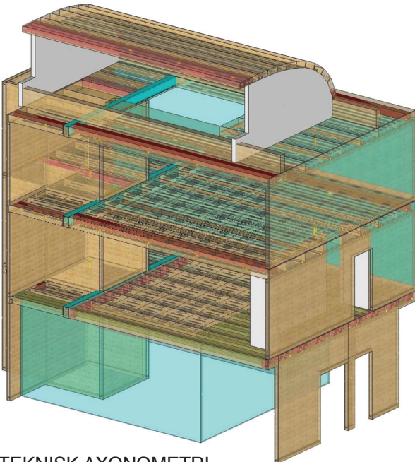
TEKNISK AXONOMETRI
