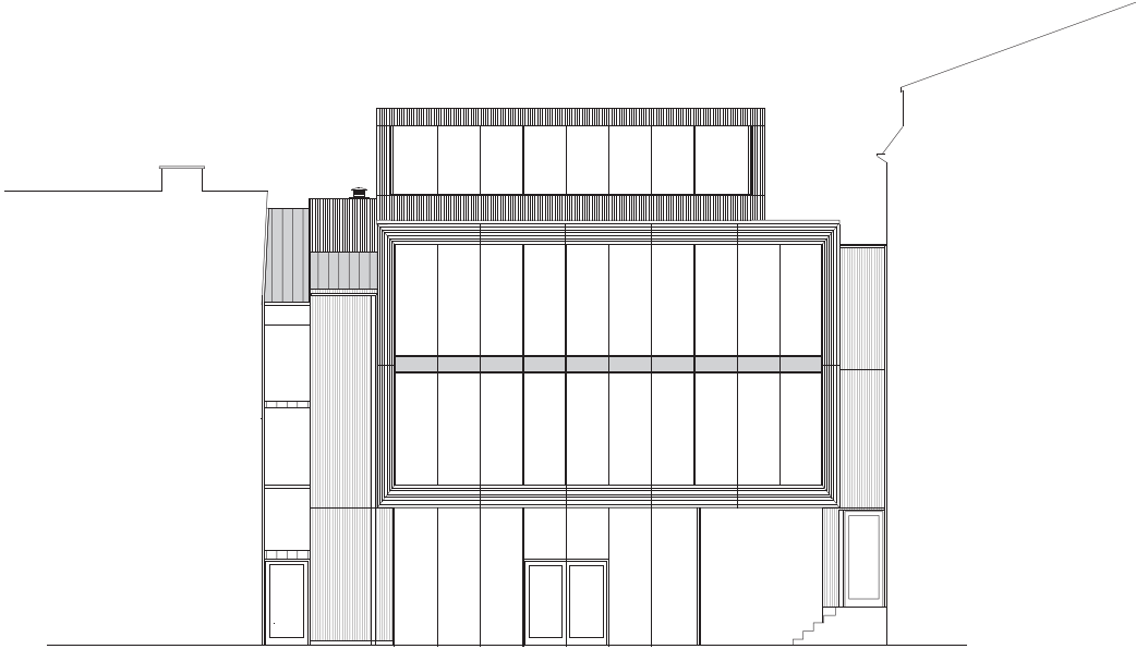
FASAD MOT ÖSTER, GÅRDEN
